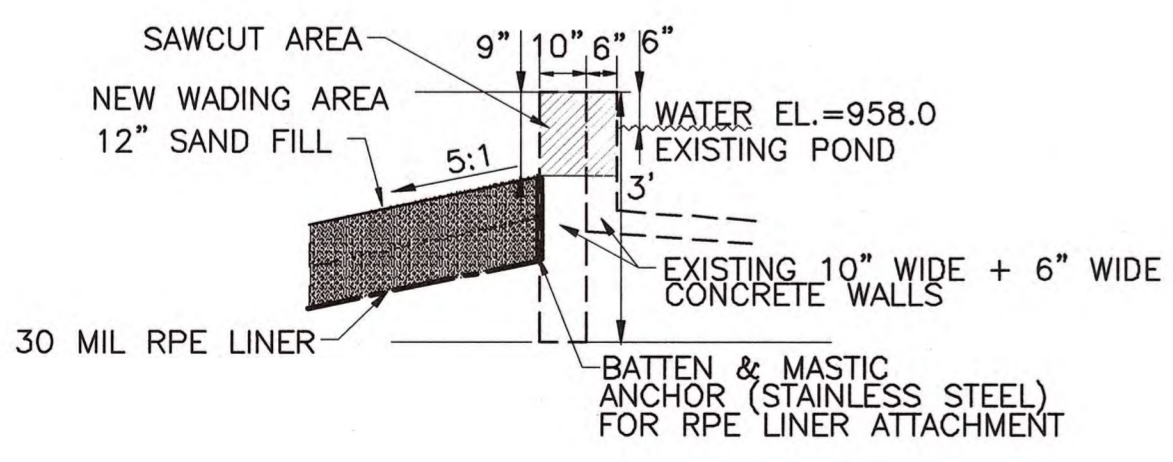
(D) SAWCUT DETAIL
