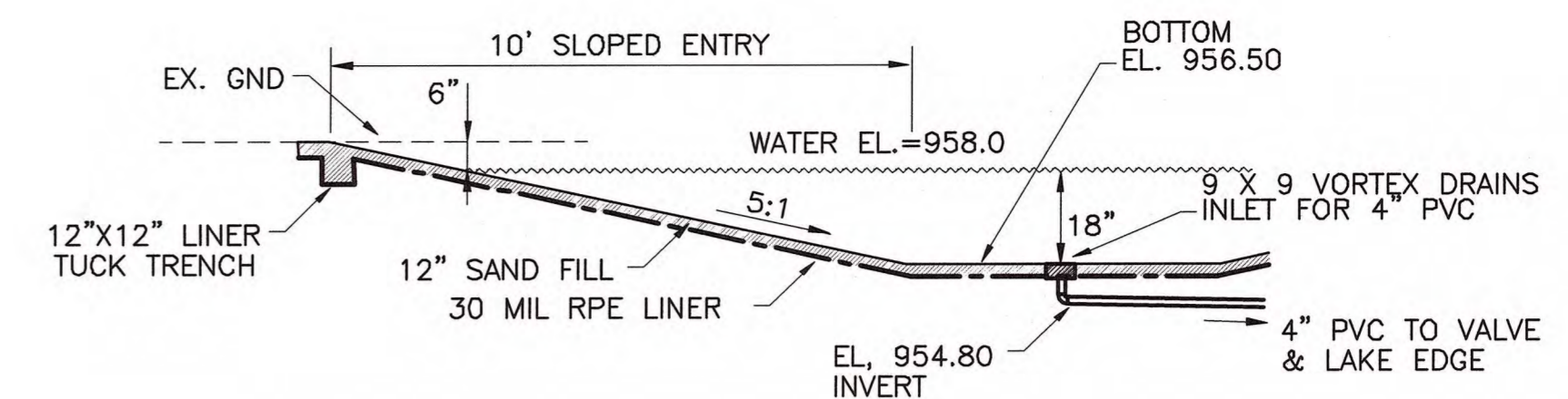
(A) NEW EDGE @ NEW WADING AREA SECTION A-A'
